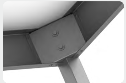
liaison solide du plan du travail avec les pieds
