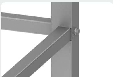
système de liaison de piètement à renfort inférieur
